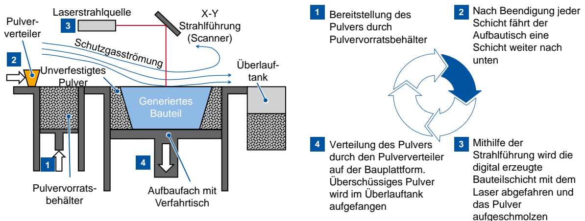
Abb. 1: Schematische Darstellung des LPBF-Prozesses angelehnt an [7]
