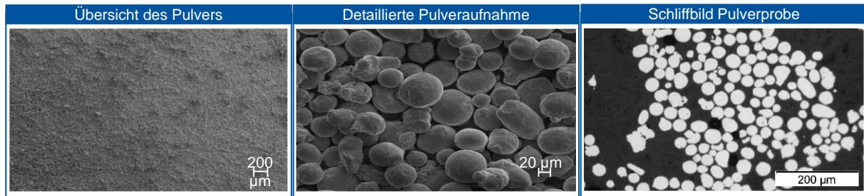
Abb. 5: Pulveraufnahmen
